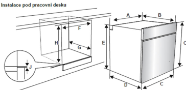
Instalace pod pracovní desku
