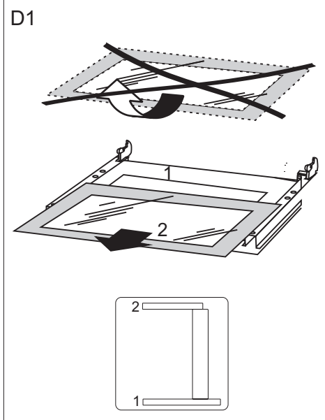
Vybratie vnútornej sklenenej tabule, dve sklá.
